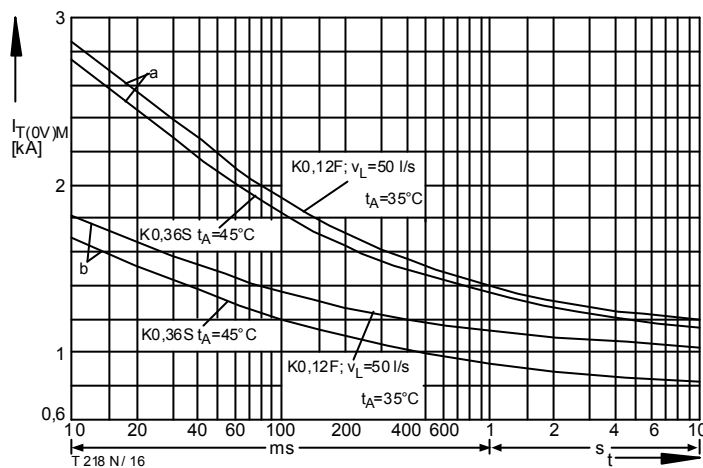
Bild / Fig. 16 Grenzzstrom / Max. overload on-state current I_{T(OV)M} = f(t) , v_{RM} = 0,8 V_{RRM} Luftselbstkühlung / Natural air-cooling, t_A = 45^\circ\text{C} Verstärkte Luftkühlung / Forced air-cooling, t_A = 35^\circ\text{C} Kühlkörper / Heatsink: K0,36S, K0,12F Belastung aus / Surge current occurs: a - Leerlauf / No-load conditions b - Betrieb mit Dauerrenzstrom / During operation at max. average on-state current I_{TAVM}
